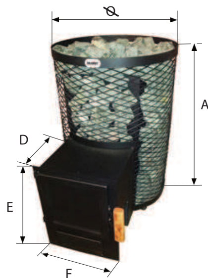
Piiirros 12. / Drawing 12. SY-216, SY-220
