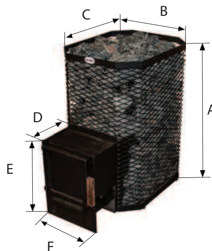
Piiirros 10. / Drawing 10. S-216, S-220
