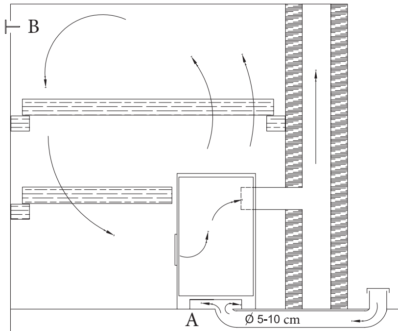
Piirros 1. Luonnollinen ilmanvaihto Drawing 1. Natural Ventilation
